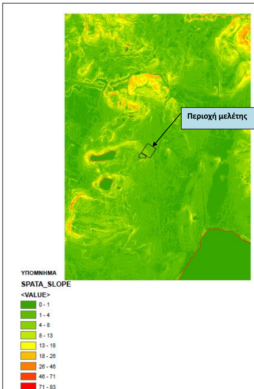
Εικόνα 2.1: Μορφολογικές κλίσεις ευρύτερης περιοχής μελέτης
