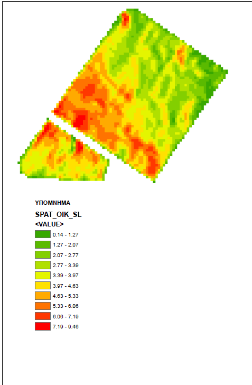
Εικόνα 2.2: Μορφολογικές κλίσεις της υπό μελέτη οικοπεδικής έκτασης
