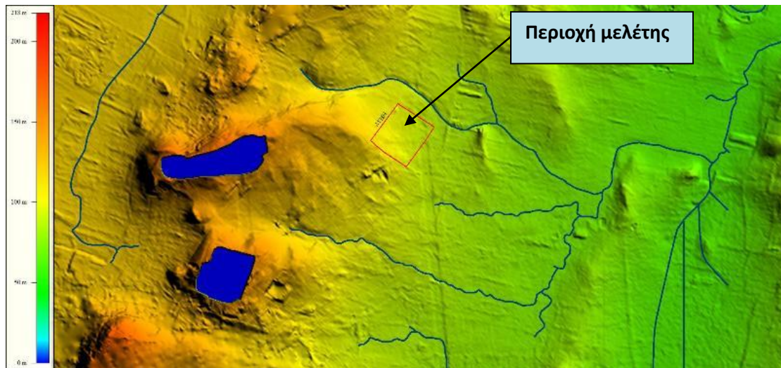
Εικόνα 2.3: Ψηφιακό ανάγλυφο της ευρύτερης περιοχής μελέτης
