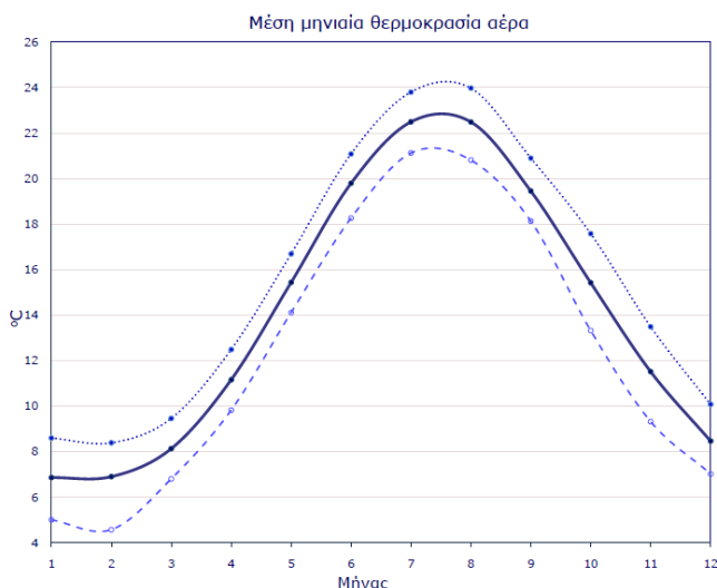
Εικόνα 4.2: Στοιχεία μέσης μηνιαίας θερμοκρασίας αέρα σταθμού EMY Ελληνικό
