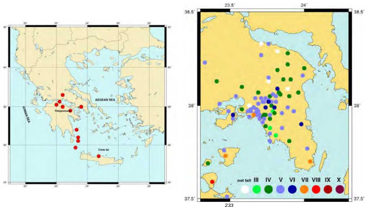
Εικόνα 6.6: Χάρτες χωρικής κατανομής των επικέντρων σεισμών με εστιακό βάθος h > 50\text{km} , για τους οποίους υπάρχουν μακροσεισμικές παρατηρήσεις για την περιοχή της Αθήνας (αριστερά) και των αντίστοιχων μέγιστων μακροσεισμικών εντάσεων κατά θέση (δεξιά). Η διαφοροποίηση στο νότιο τμήμα του νομού σε σχέση με το
