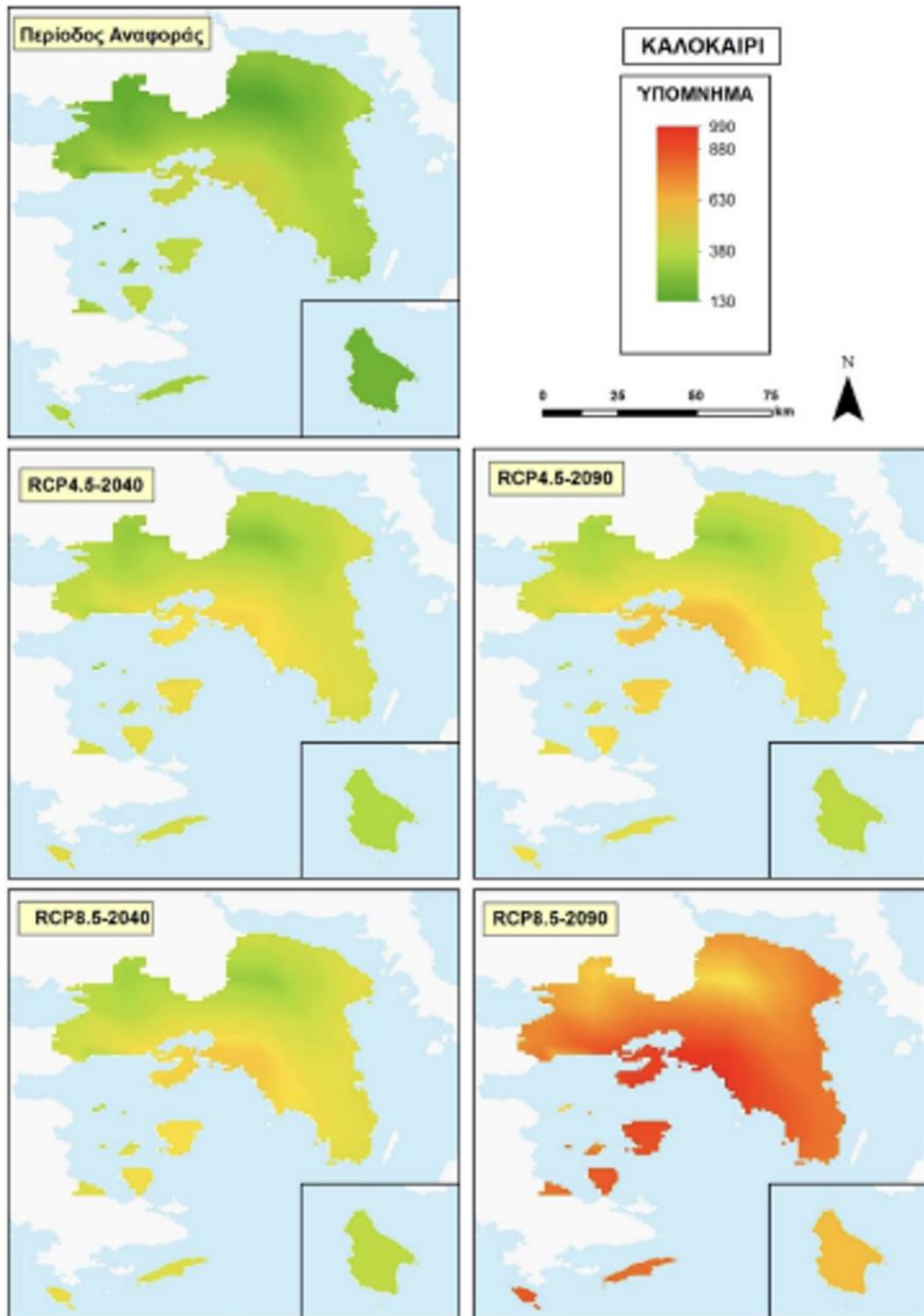
Εικόνα 65 Βαθμομέρες ψύξης – Θέρος
