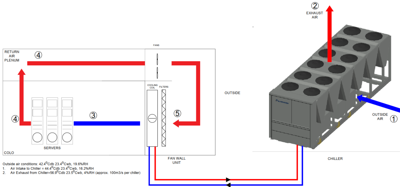
Εικόνα 39 Σύστημα αέρα-νερού με αερόψυκτους ψύκτες
