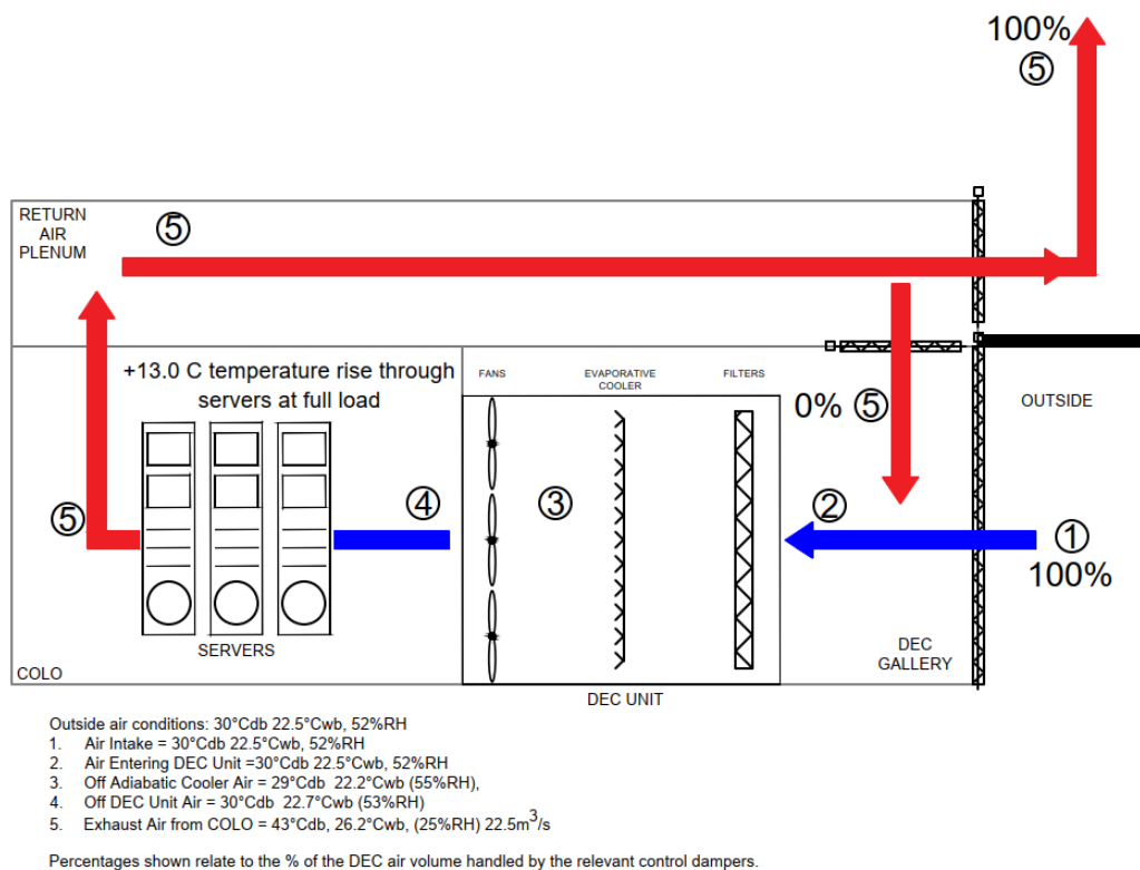
Εικόνα 28 Λειτουργία εξατμιστικής ψύξης.
