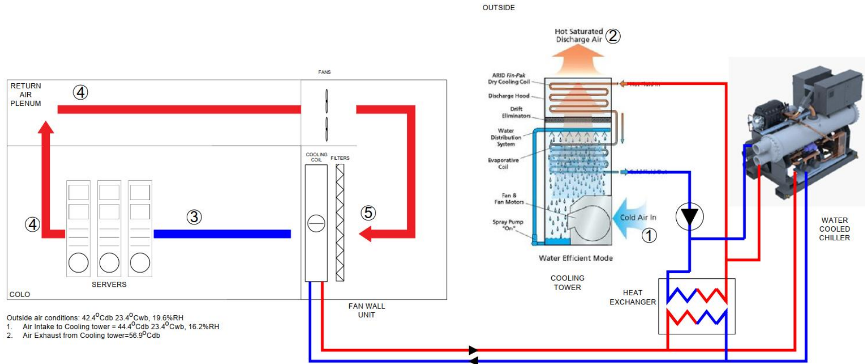
Εικόνα 40 Υβριδικό σύστημα ψύξης αέρα-νερού με υδρόψυκτους ψύκτες και πύργους ψύξης
