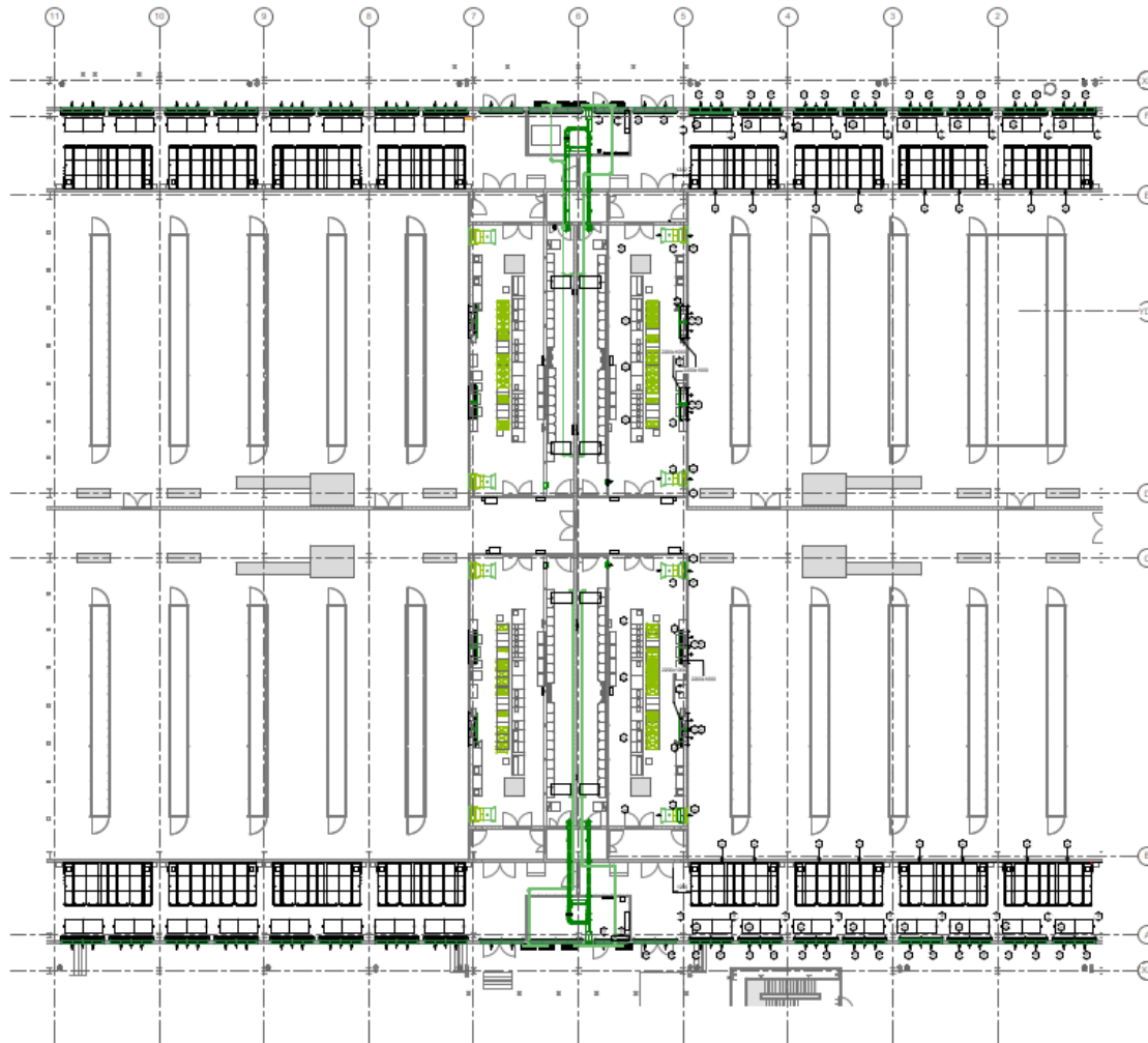
Εικόνα 23 Διάταξη του συστήματος ψύξης σε ένα Colo.
