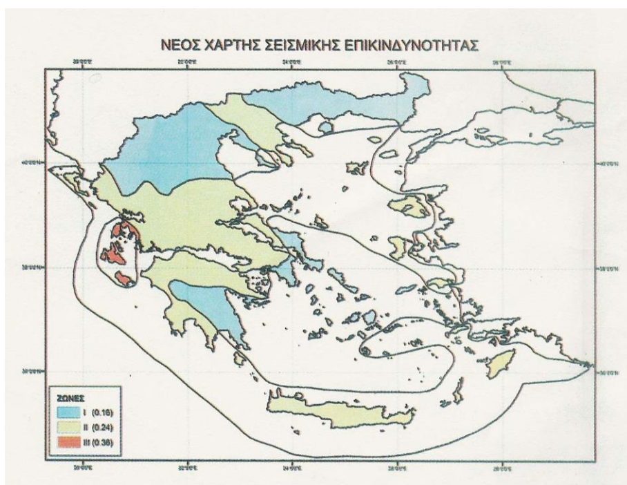
Εικόνα 75 Χάρτης σεισμικής επικινδυνότητας
