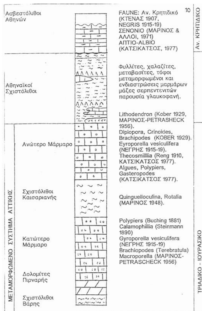
Εικόνα 71 Σχηματική στρωματογραφική κολώνα της ζώνης Αττικής
