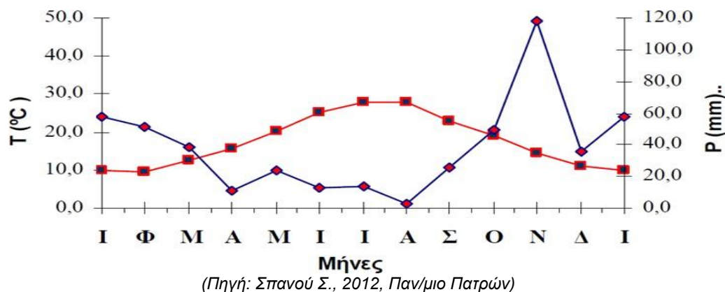
Εικόνα 51 Ομβροθερμικό διάγραμμα ΜΣ Σπάτων.
