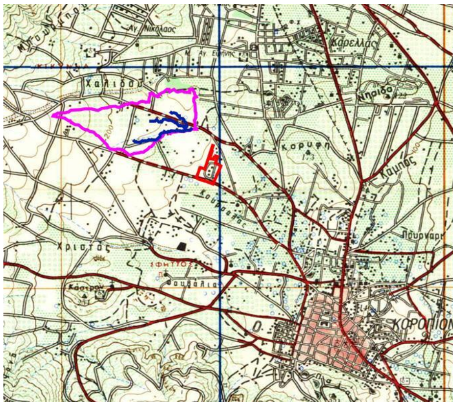
Εικόνα 106 Υδρολογική λεκάνη πλησιέστερου προς το υπό μελέτη οικόπεδο ρέματος
