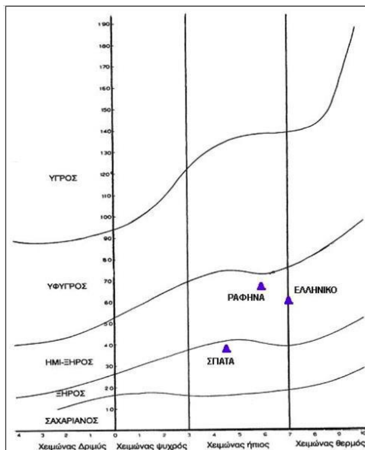
Εικόνα 49 Κλιματικό διάγραμμα Emburger Σπάτα – Ραφήνα – Ελληνικό.
