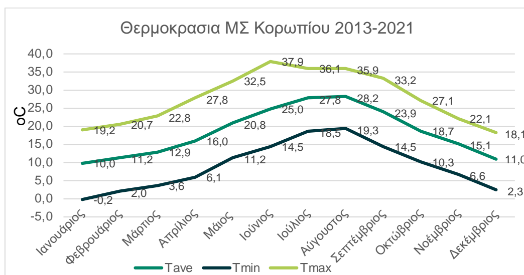
Εικόνα 40 Κατανομή μέσης, μέσης μέγιστης και μέσης ελάχιστης θερμοκρασίας ΜΣ Κορωπίου (2013 – 2021)
