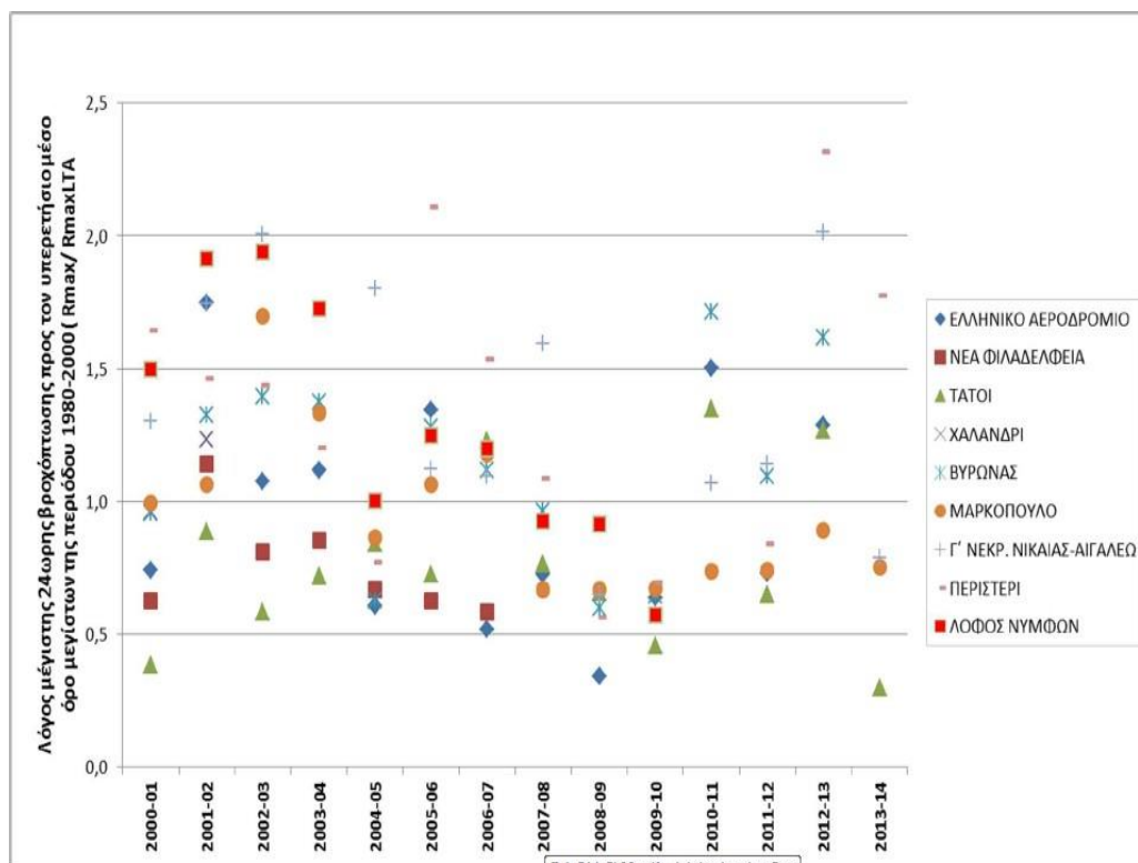
Εικόνα 111 Σχέση των μέγιστων ημερήσιων βροχοπτώσεων με τον υπερετήσιο μέσο όρο των μέγιστων ημερήσιων βροχοπτώσεων της περιόδου 1980-2000 ανά έτος και σταθμό ( R_{max} \text{ Έτους} / R_{maxLTA} ).
