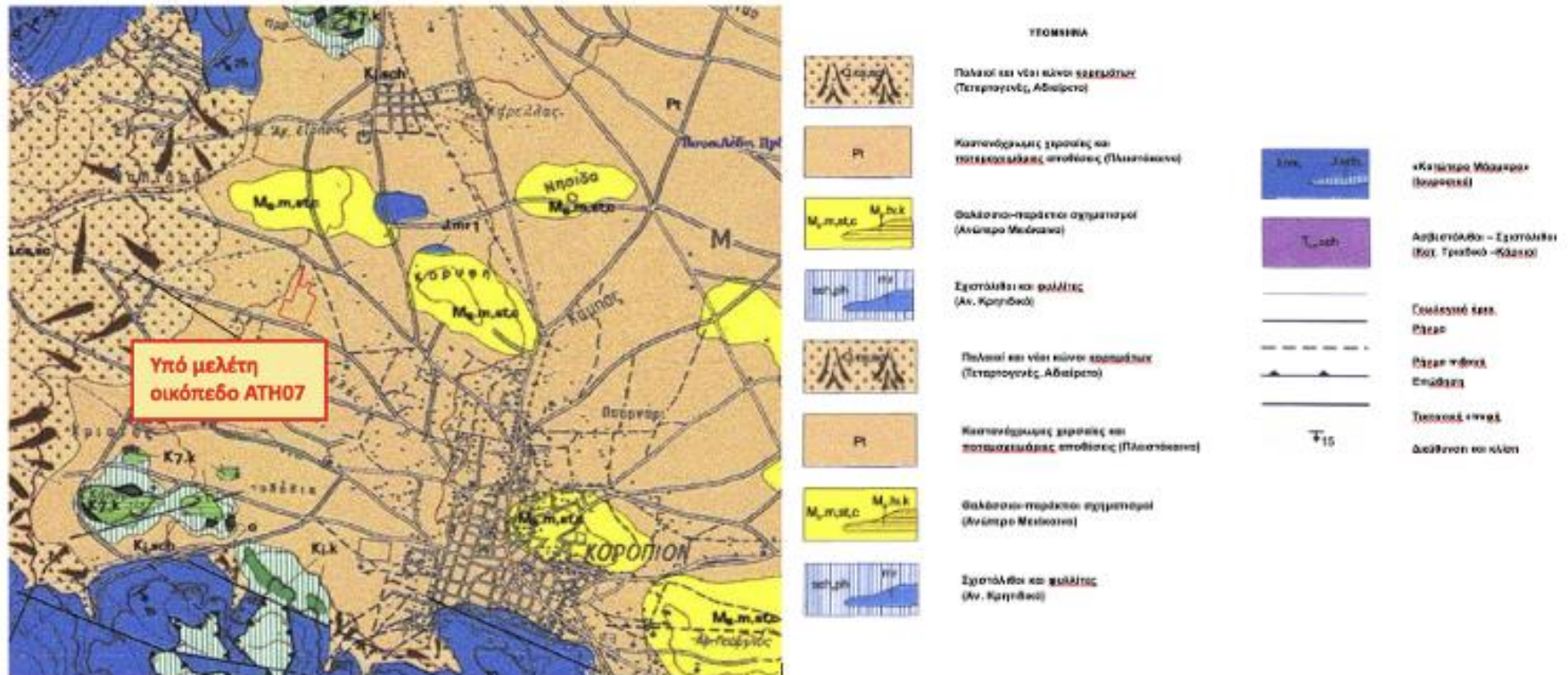
Εικόνα 72 Απόσπασμα γεωλογικού χάρτη ΙΓΜΕ με την ευρύτερη περιοχή του Κορωπίου.
