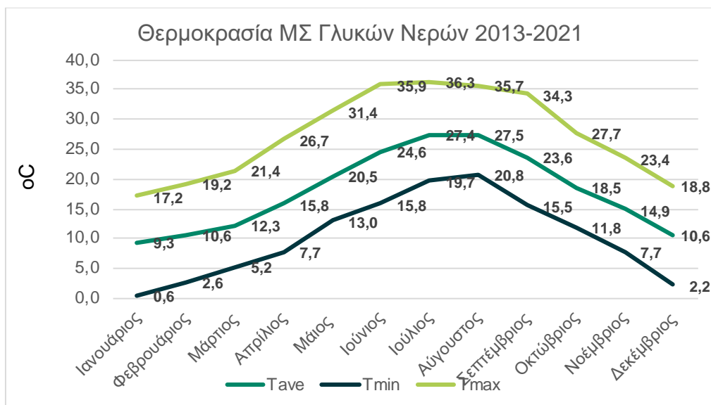
Εικόνα 41 Κατανομή μέσης, μέσης μέγιστης και μέσης ελάχιστης θερμοκρασίας ΜΣ Γλυκών Νερών (2013 – 2021)
