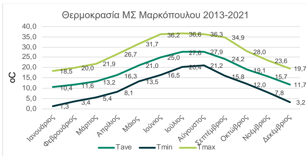
Εικόνα 42 Κατανομή μέσης, μέσης μέγιστης και μέσης ελάχιστης θερμοκρασίας ΜΣ Μαρκόπουλου (2013 – 2021)
