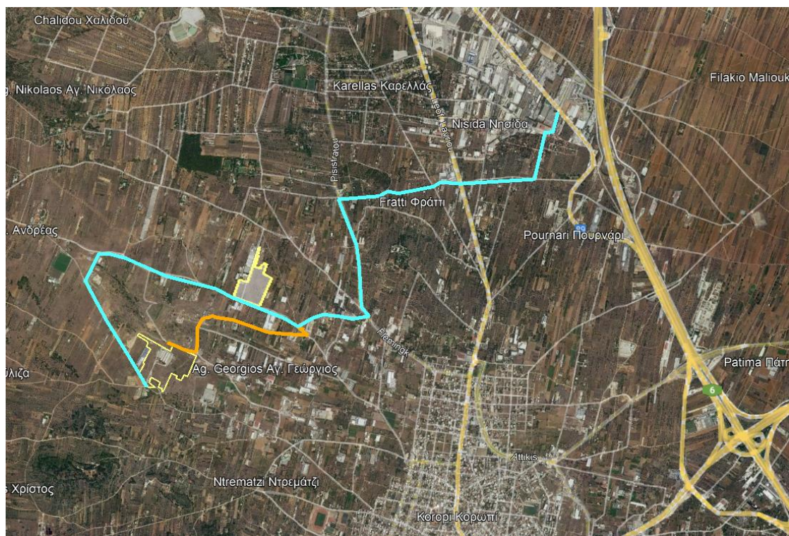
Εικόνα 30 Δίκτυο ύδρευσης και θέση οικοπέδου - Προκαταρκτική προσέγγιση όδευσης – Εναλλακτική 2
