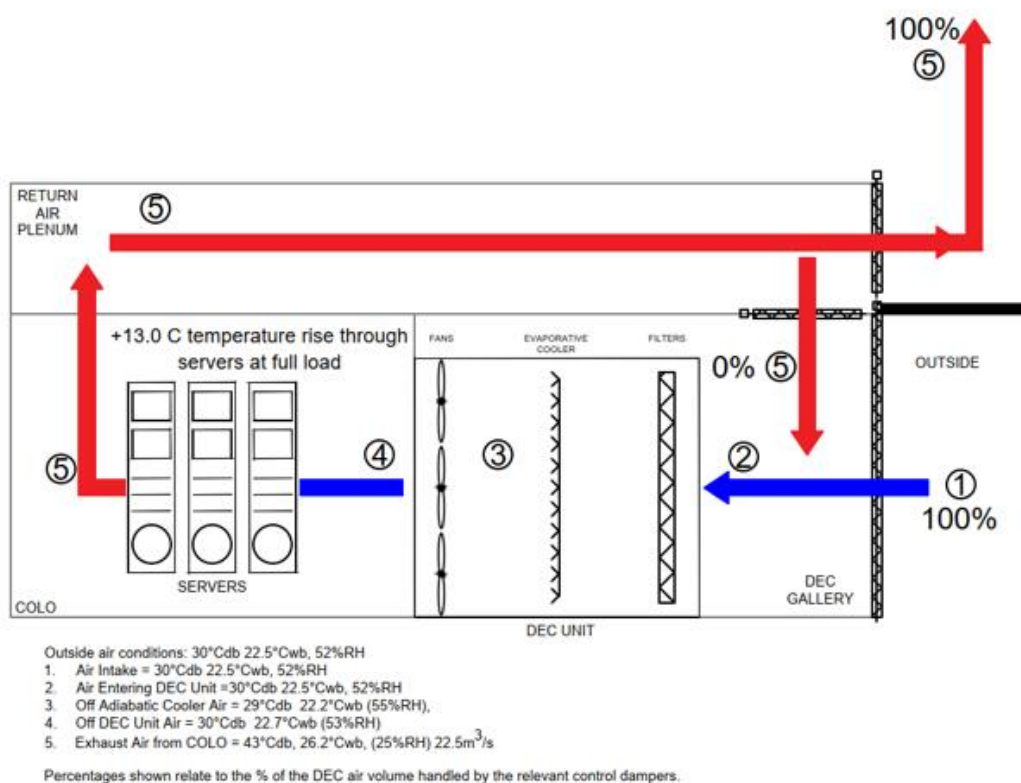
Εικόνα 26 Λειτουργία εξατμιστικής ψύξης.
