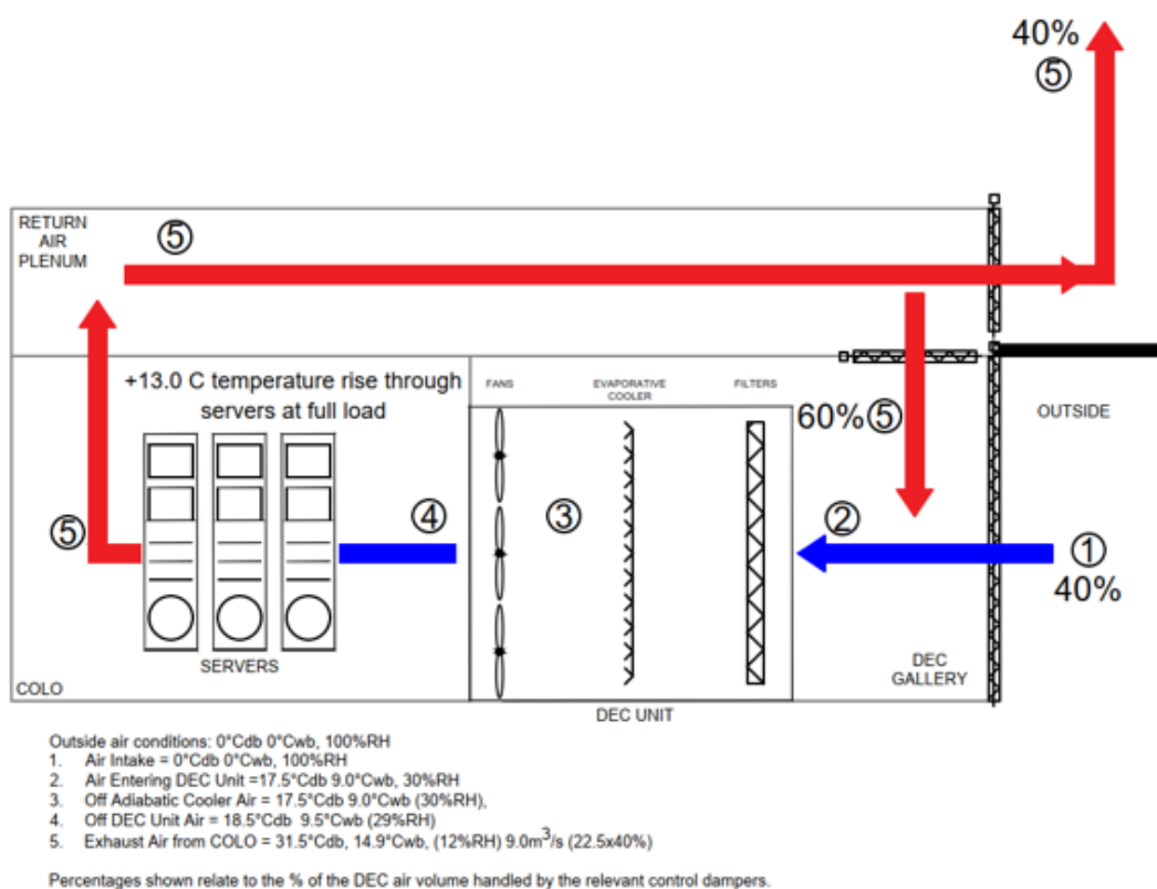
Εικόνα 24 Συνθήκες λειτουργία συστήματος προσαγωγής, για εξωτερική θερμοκρασία 0 °C DB
