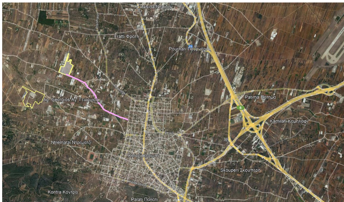
Εικόνα 28 Δίκτυο αποχέτευσης και η θέση του οικοπέδου ATH07 - Προκαταρκτική προσέγγιση όδευσης – εναλλακτική 2
