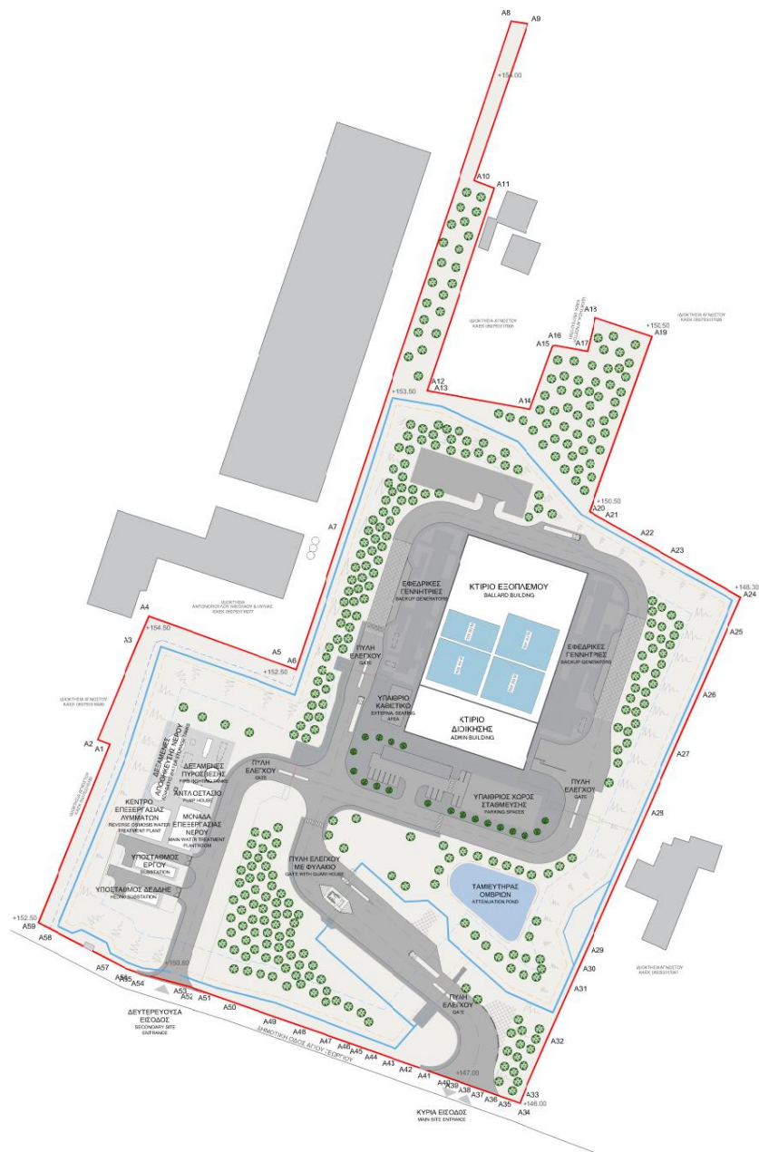
Εικόνα 17 Master plan του έργου με ενσωματωμένα τα νέα κτήρια και τις εγκαταστάσεις
