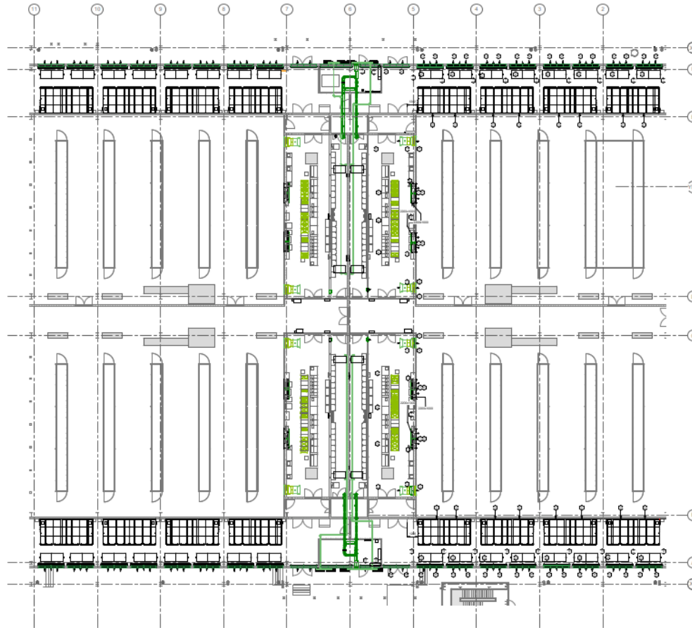
Εικόνα 21 Διάταξη του συστήματος ψύξης σε ένα Colo.
