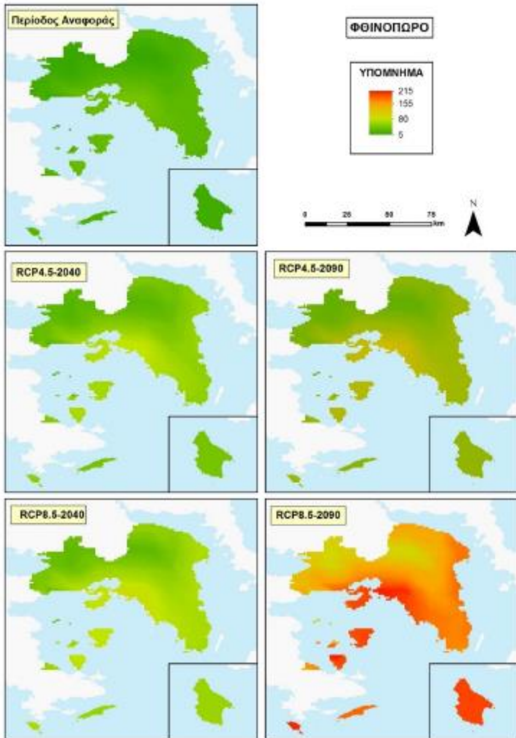
Εικόνα 68 Βαθμομέρες ψύξης – Φθινόπωρο
