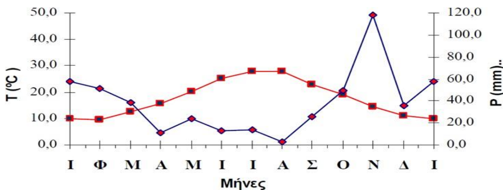
Εικόνα 52 Ομβροθερμικό διάγραμμα ΜΣ Σπάτων
