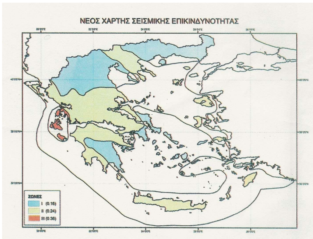
Εικόνα 76 Χάρτης σεισμικής επικινδυνότητας.
