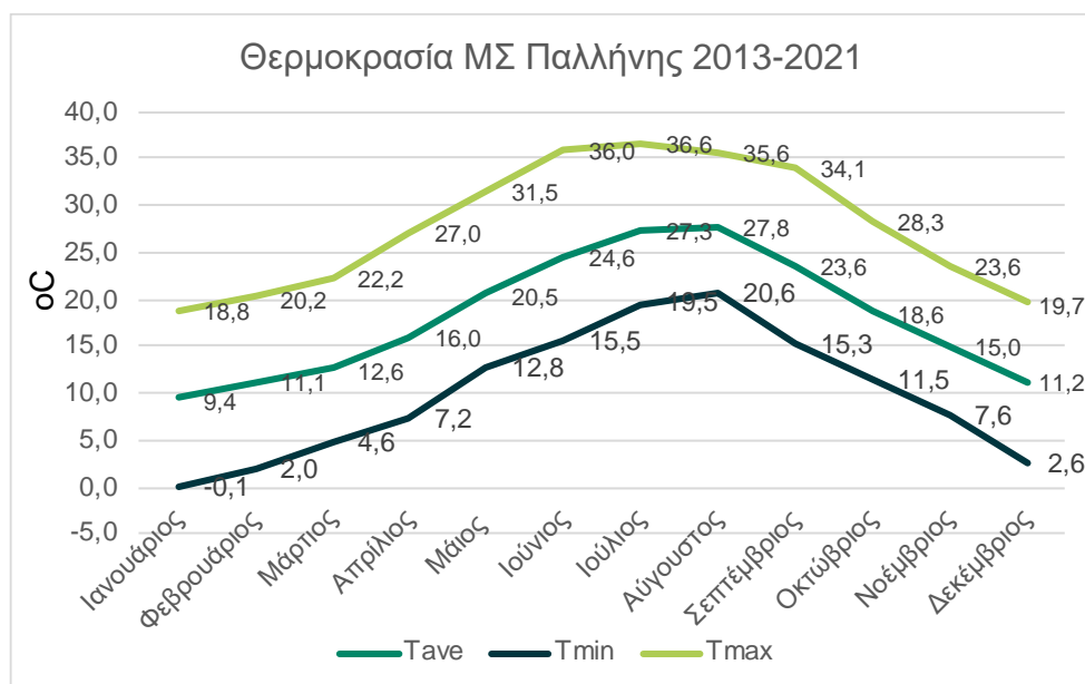
Εικόνα 44 Κατανομή μέσης, μέσης μέγιστης και μέσης ελάχιστης θερμοκρασίας ΜΣ Παλλήνης (2013 – 2021)
