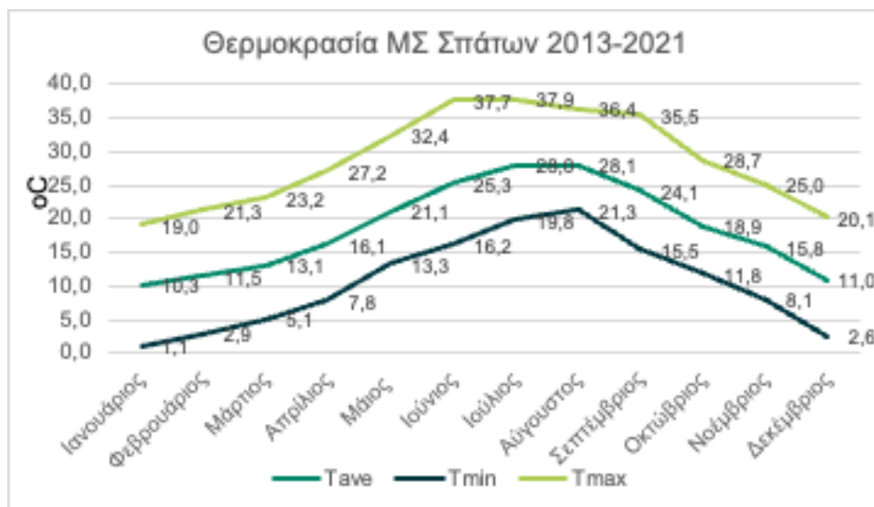
Εικόνα 43 Κατανομή μέσης, μέσης μέγιστης και μέσης ελάχιστης θερμοκρασίας ΜΣ Σπάτων (2013 – 2021)
