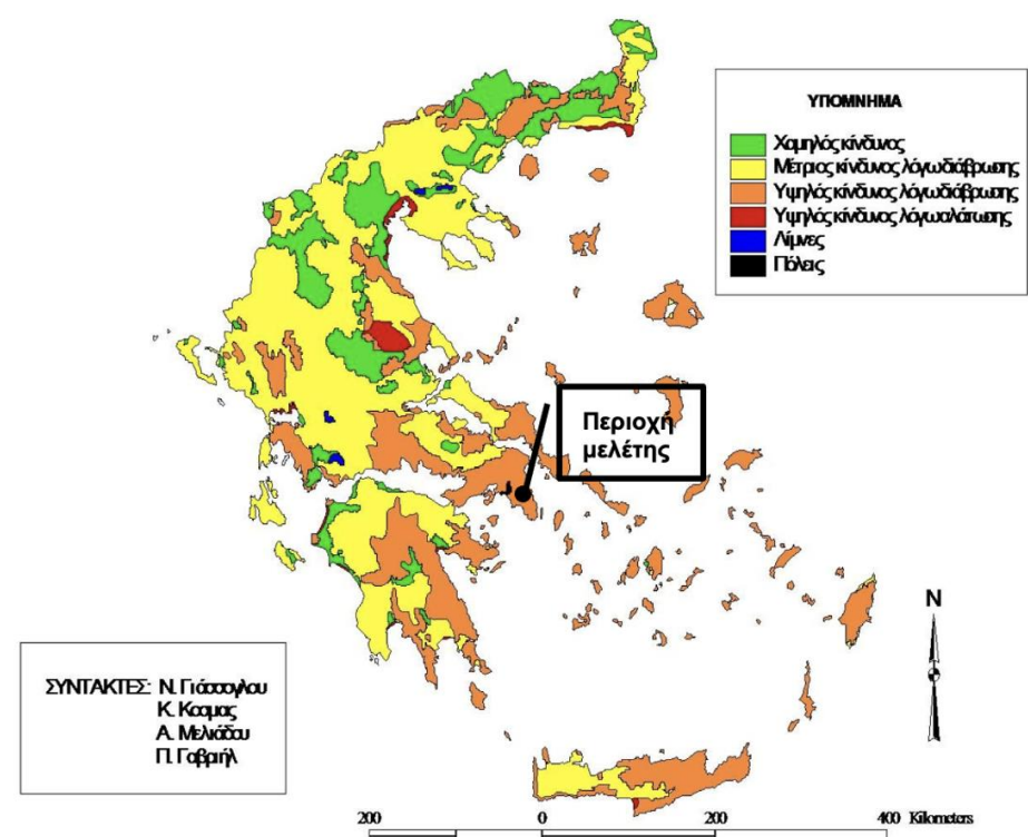
Εικόνα 100 Χάρτης δυνητικού κινδύνου ερημοποίησης της Ελλάδας (Εθνική Επιτροπή κατά της Ερημοποίησης).
